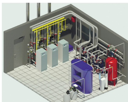
3D-визуализация предпроектного решения котельной мощностью 750 кВт
